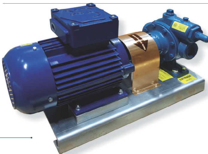
Grupo de bombeo de 1.000 L/min. para cargaderos de camiones cisterna, instalaciones industriales y repostado de gran caudal.
